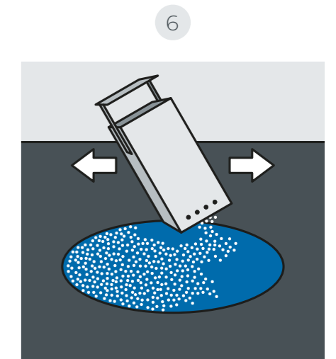
SWARCO PREFORMED Playground mit Nachstreumittel abstreuen.
