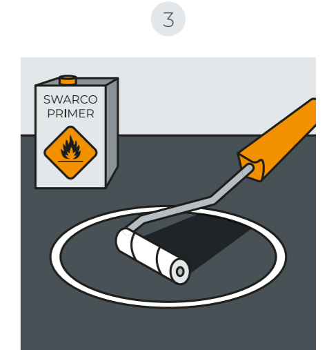
Untergrund bei Kälte und Nässe gründlich vorwärmen bzw. vortrocknen. Grundierung auftragen und ablüften lassen.
